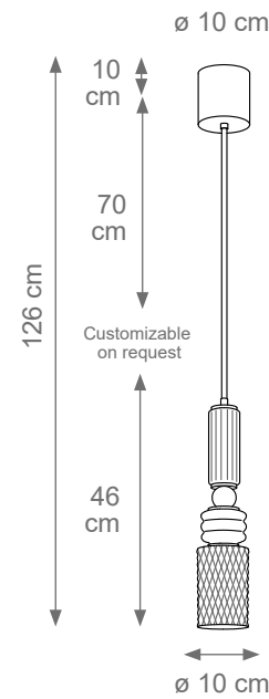
Fifi Pendant Light Code F808109 Type 1 light electrification x Max 28W E14 CE Size: cm. 46 h x 10 ø - 1,2 kg
