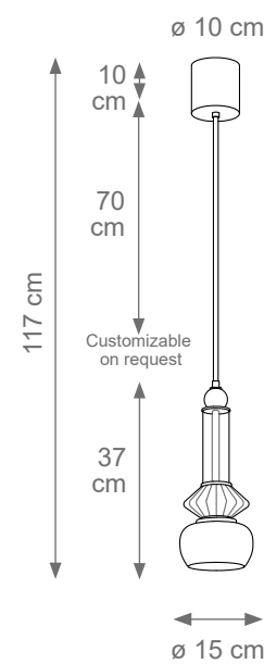
Marie Pendant Light Code F808111 Type 1 light electrification x Max 28W E14 CE Size: cm. 37 h x 15 ø - 1,1 kg
