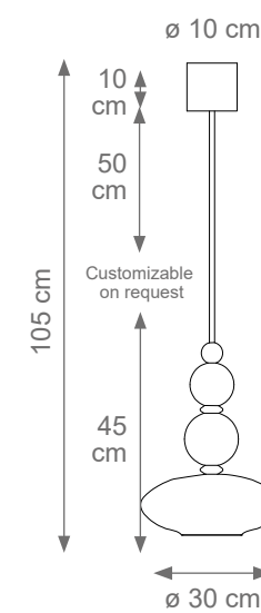
Rita Pendant Light Code F807345 Type 1 light electrification x Max 28W E14 CE Size: cm. 45 h x 30 ø - 3 kg
