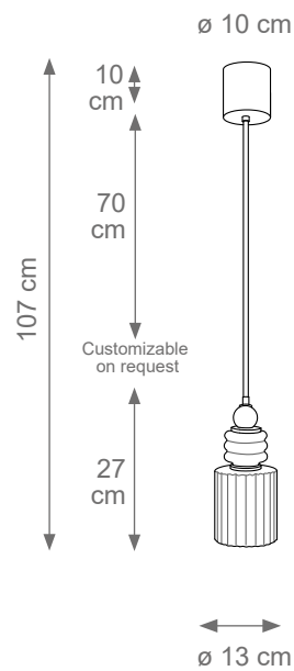
Silvy Pendant Light Code F808112 Type 1 light electrification x Max 28W E14 CE Size: cm. 27 h x 13 ø - 1 kg
