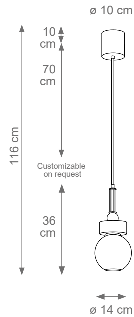
Etienne Pendant Light Code F808108 Type 1 light electrification x Max 28W E14 CE Size: cm. 36 h x 16 ø - 2,2 kg
