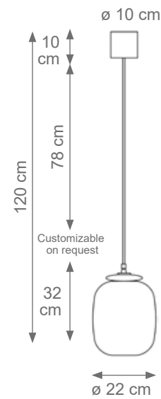
Soho Pendant Light Code: F808031 Type 1 light electrification x Max 28W E14 CE Size: cm. 32 h x 22 ø - 2,5 kg
