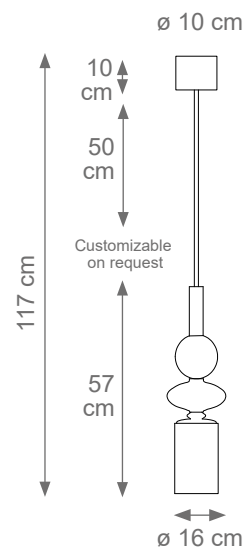
Greta Pendant Light Code F807342 Type 1 light electrification x Max 28W E14 CE Size: cm. 57 h x 16 ø - 3 kg
